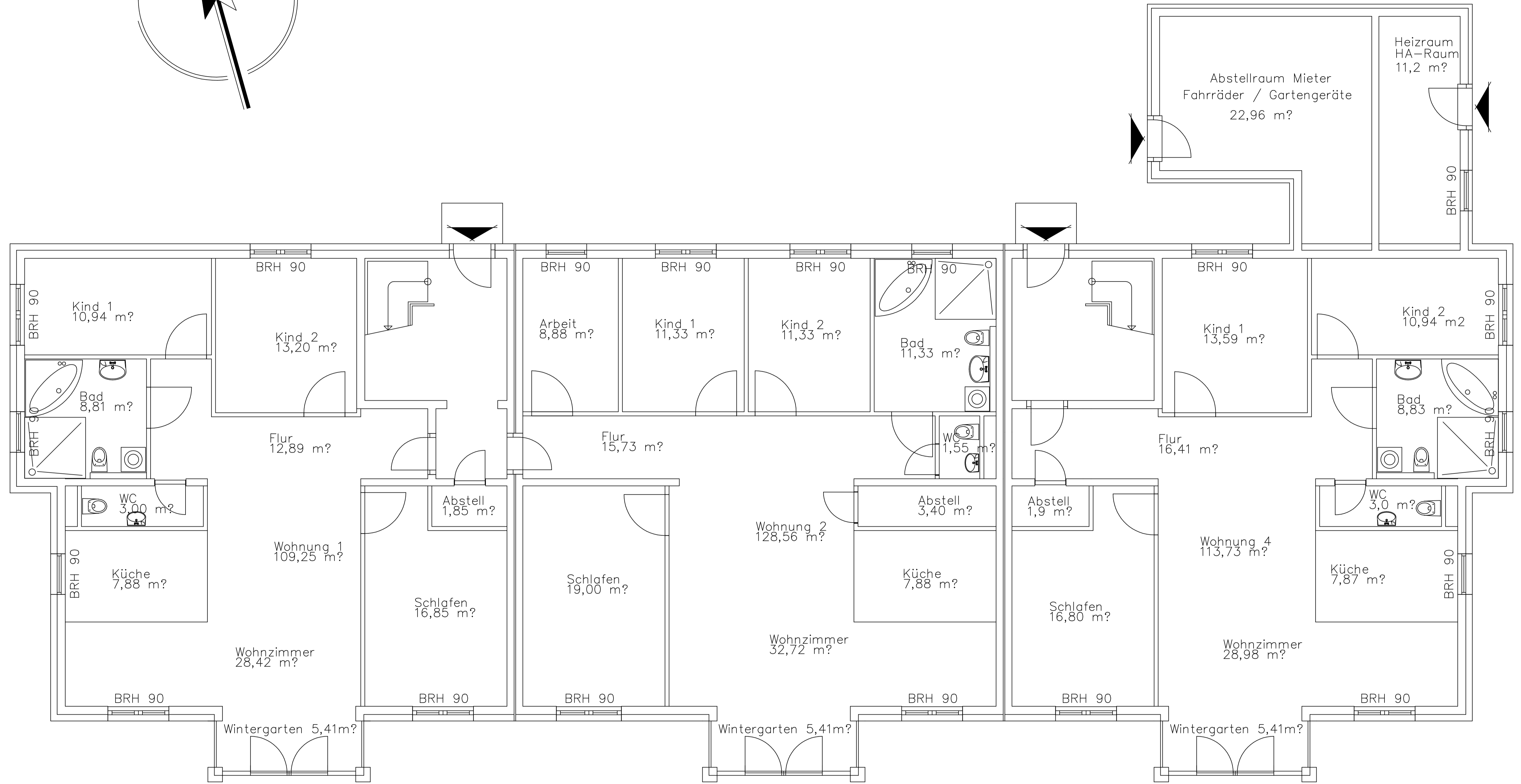
Grundriss EG
